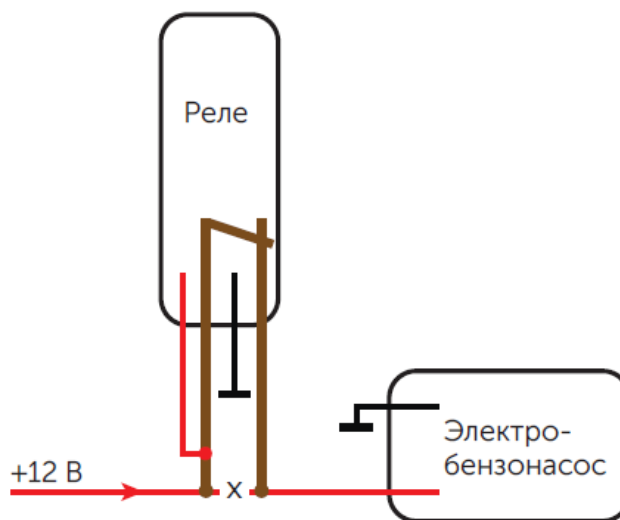
Рисунок 3 – схема подключения реле блокировки в цепь питания бензонасоса.
